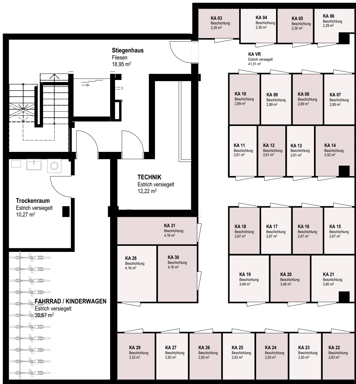
-2 KELLERABTEILE
